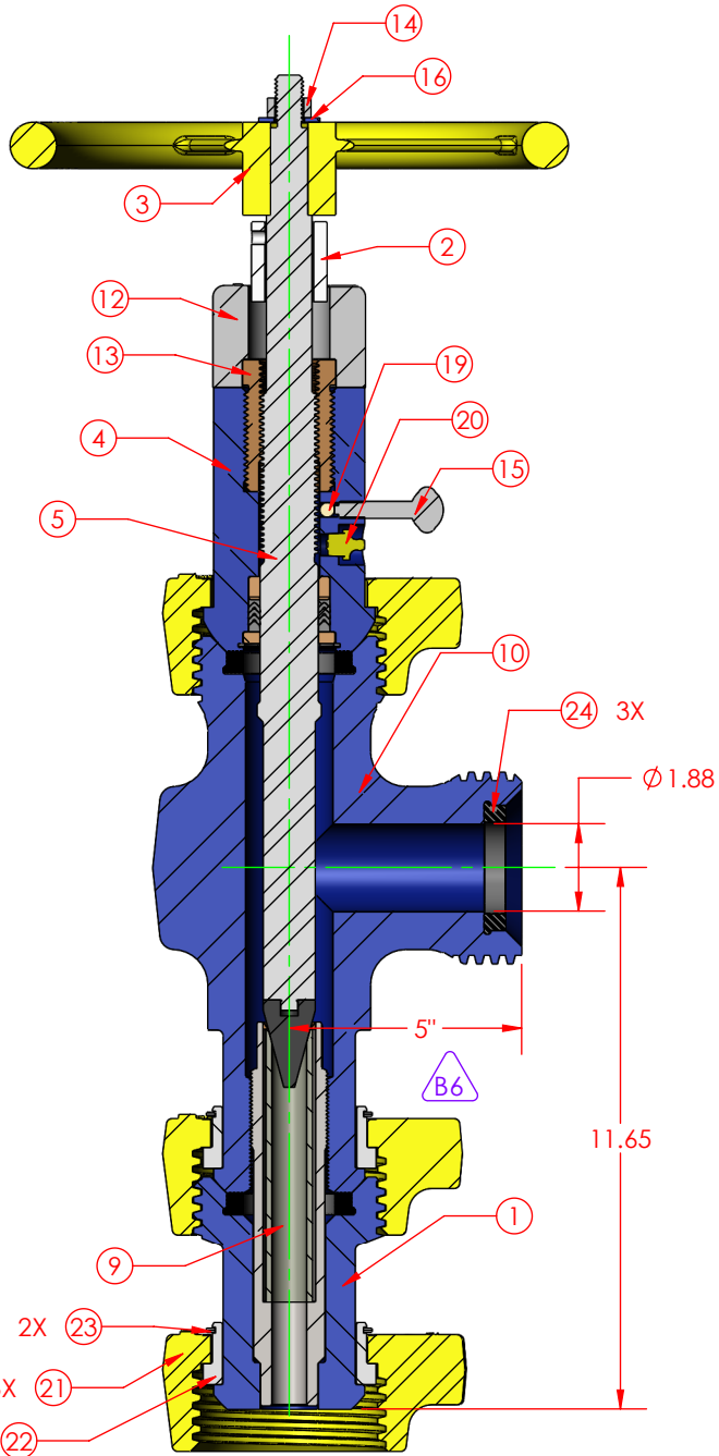
SECTION A-A
